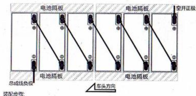
电池连接示意图
