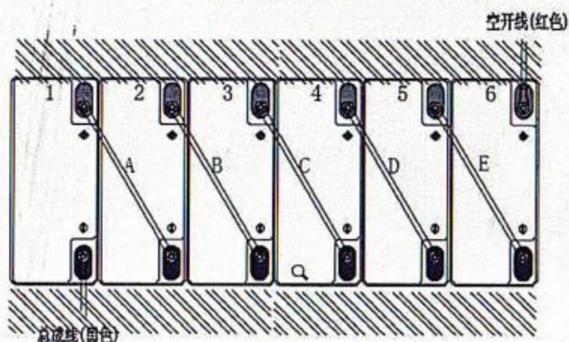
电池连接示意图
