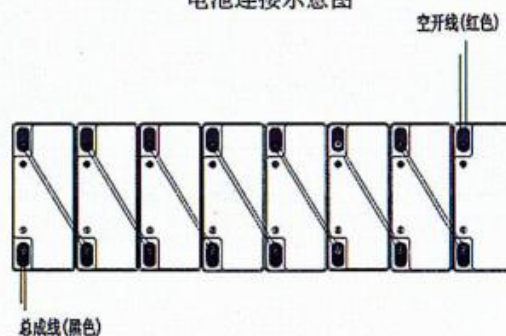
电池连接示意图
